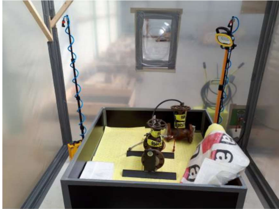
Foto 1: opstelling multitools
